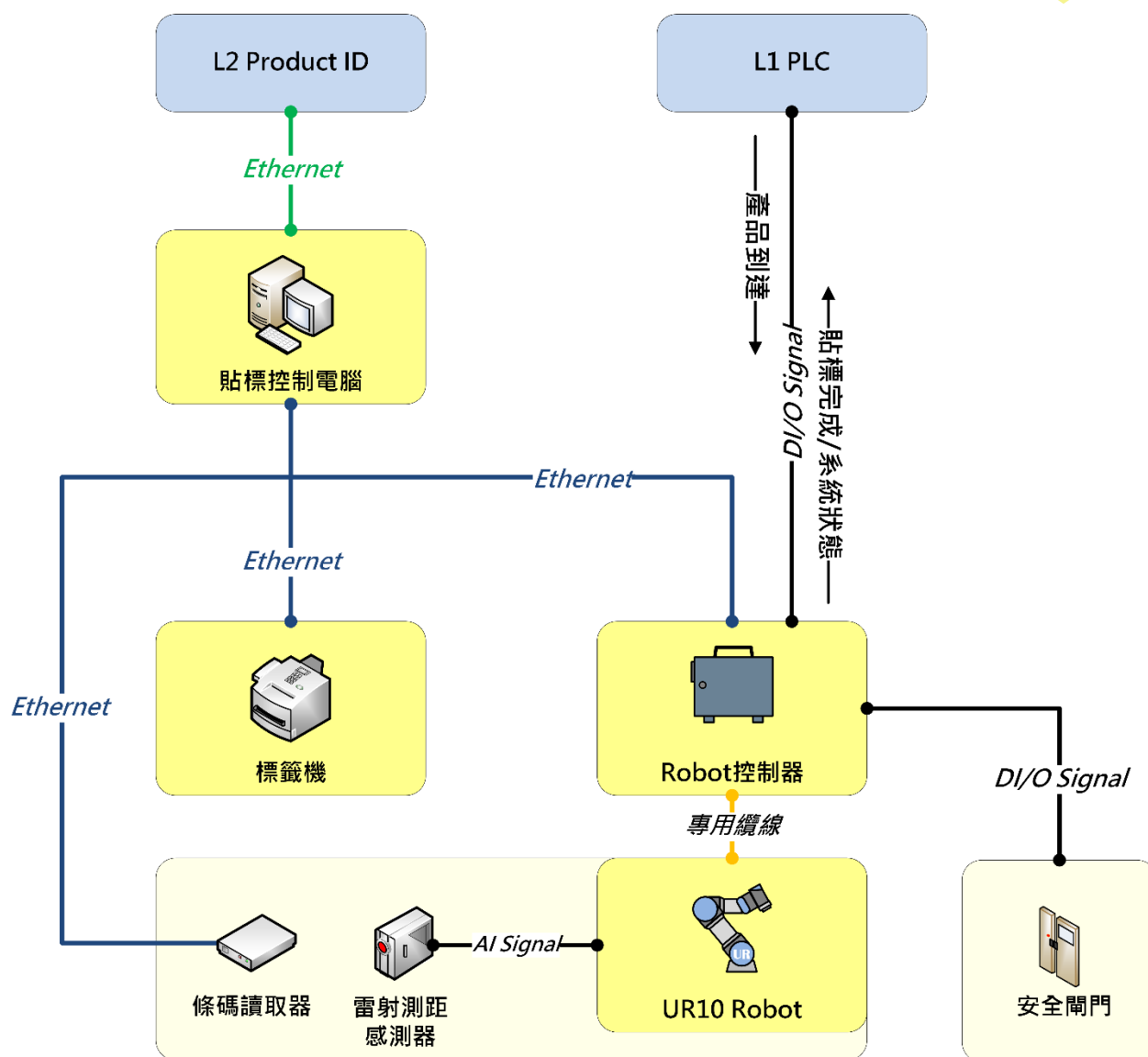
產品架構圖
