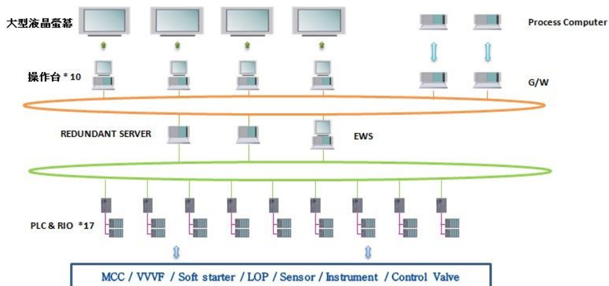
系統架構圖
