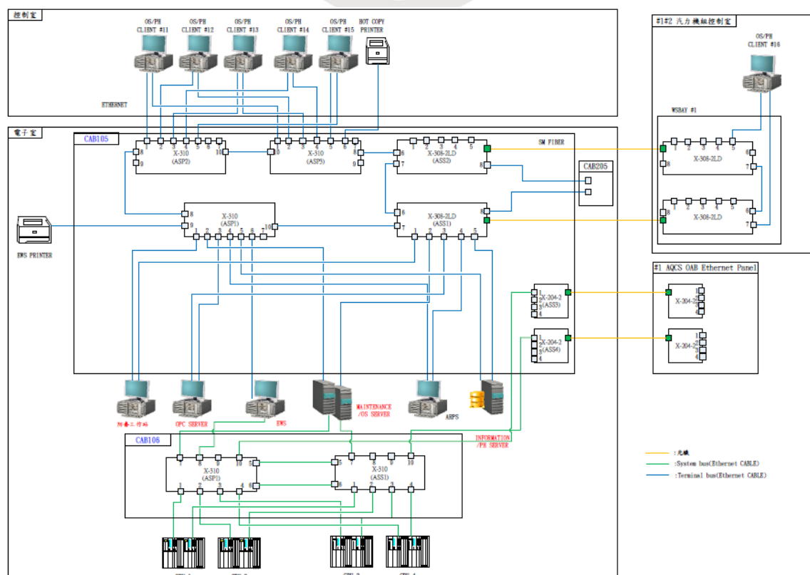
FGD 系統架構圖
