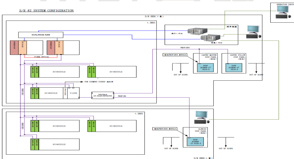
取煤機系統架構圖
