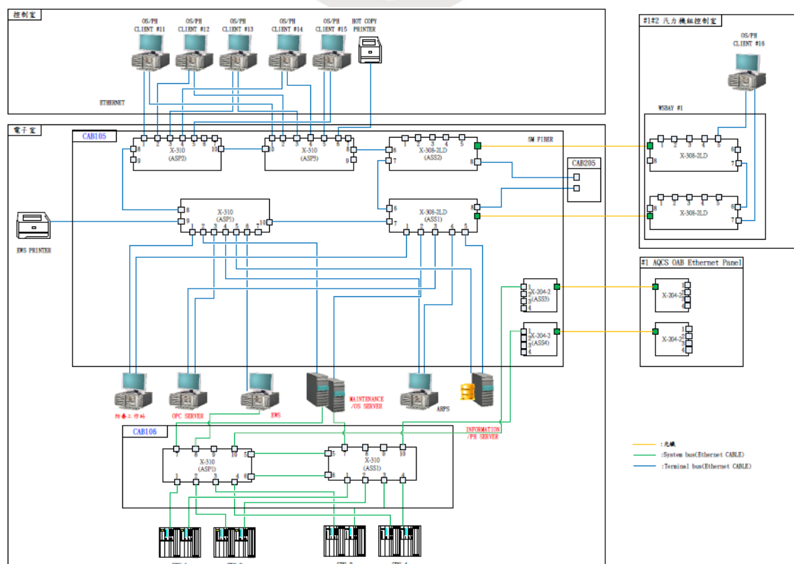
FGD 系统架构图
