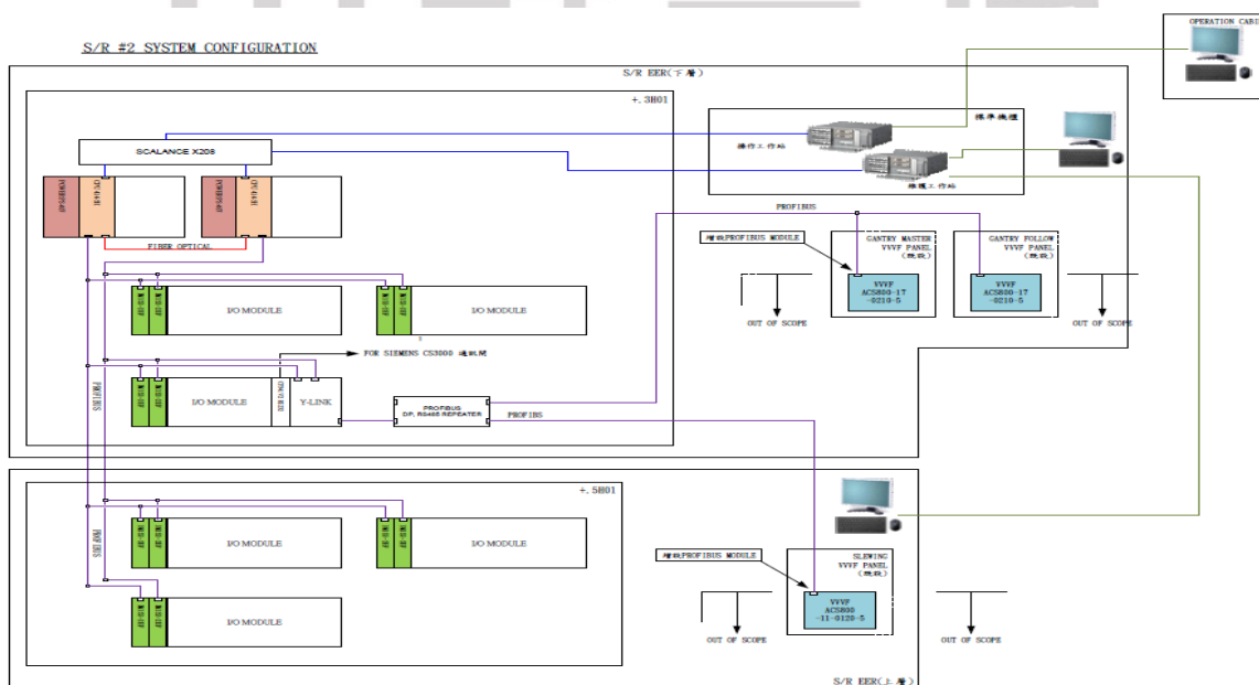
取煤机系统架构图
