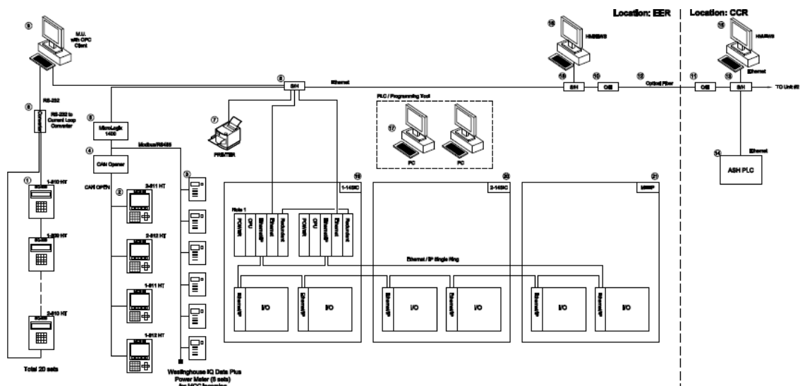
EP 系统架构图
